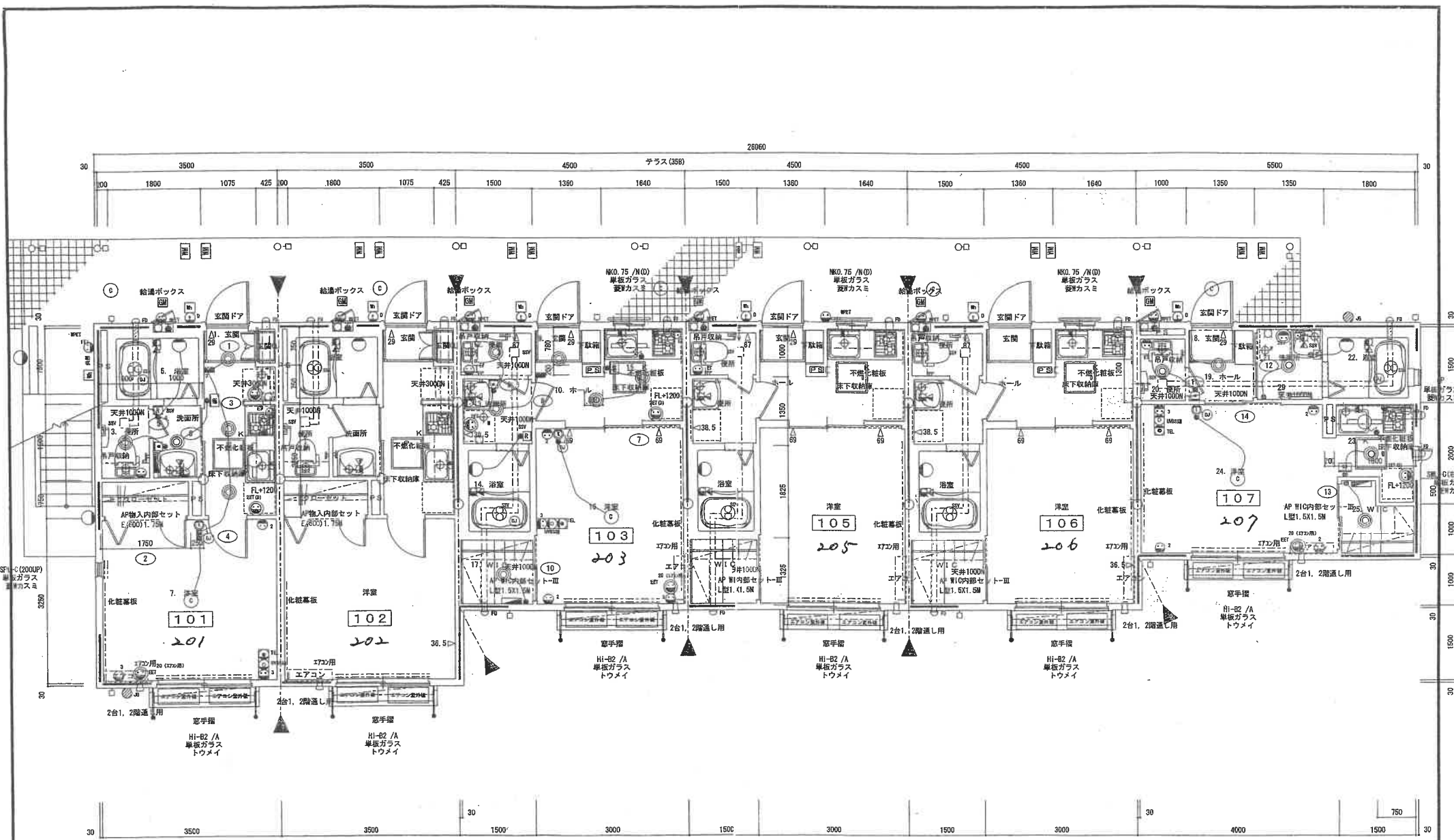
1階平面図 1/50
