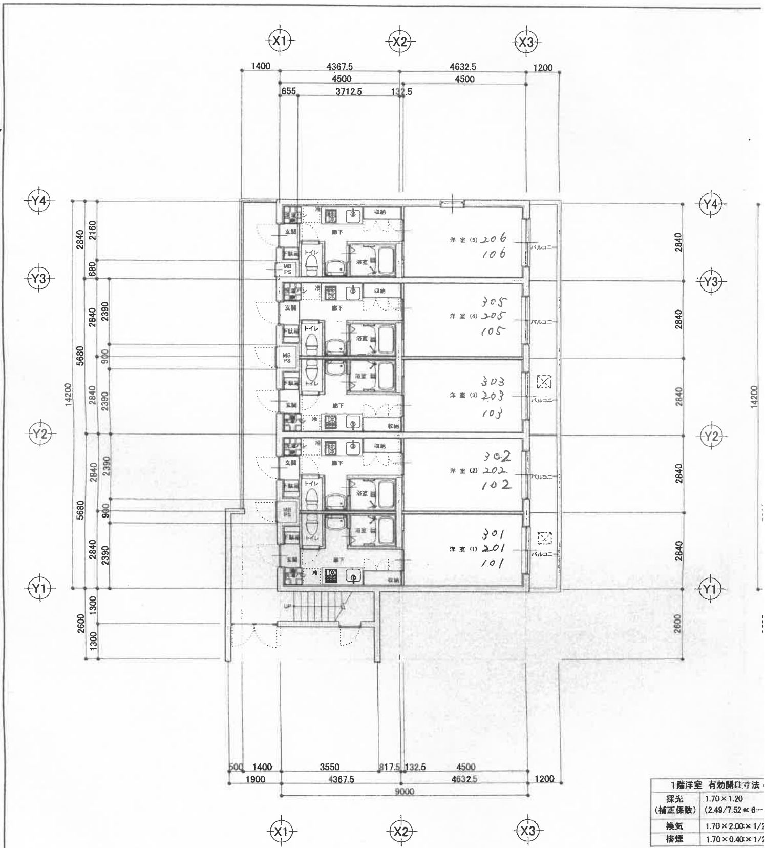
1階 平面図 S=1/100
