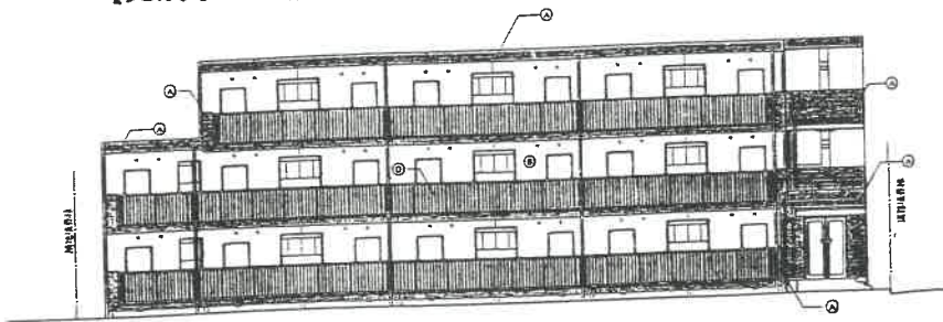
北側立面図
