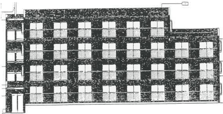
南立面图
